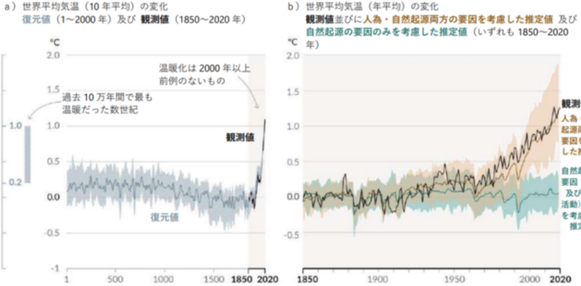
図 SPM.1：世界の気温変化の歴史と近年の昇温の原因
