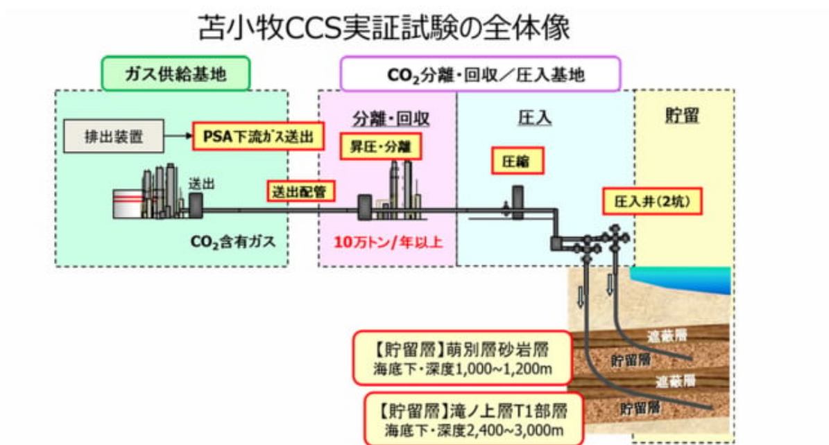
PSA（Pressure Swing Adsorption、圧カスイング吸着）： 水素製造装置の生成ガスから高純度水素ガスを得る装置。PSA装置からの下流ガスには高濃度CO 2 が含まれる。
