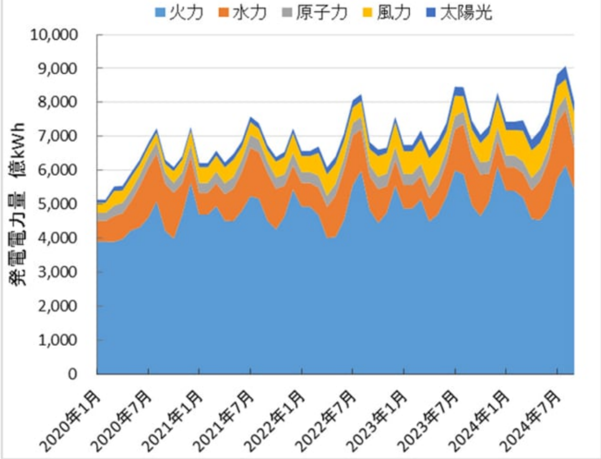
図-14 近年の中国の月間発電電力量の推移 出所: 中国国家情報局、月次報告データ
