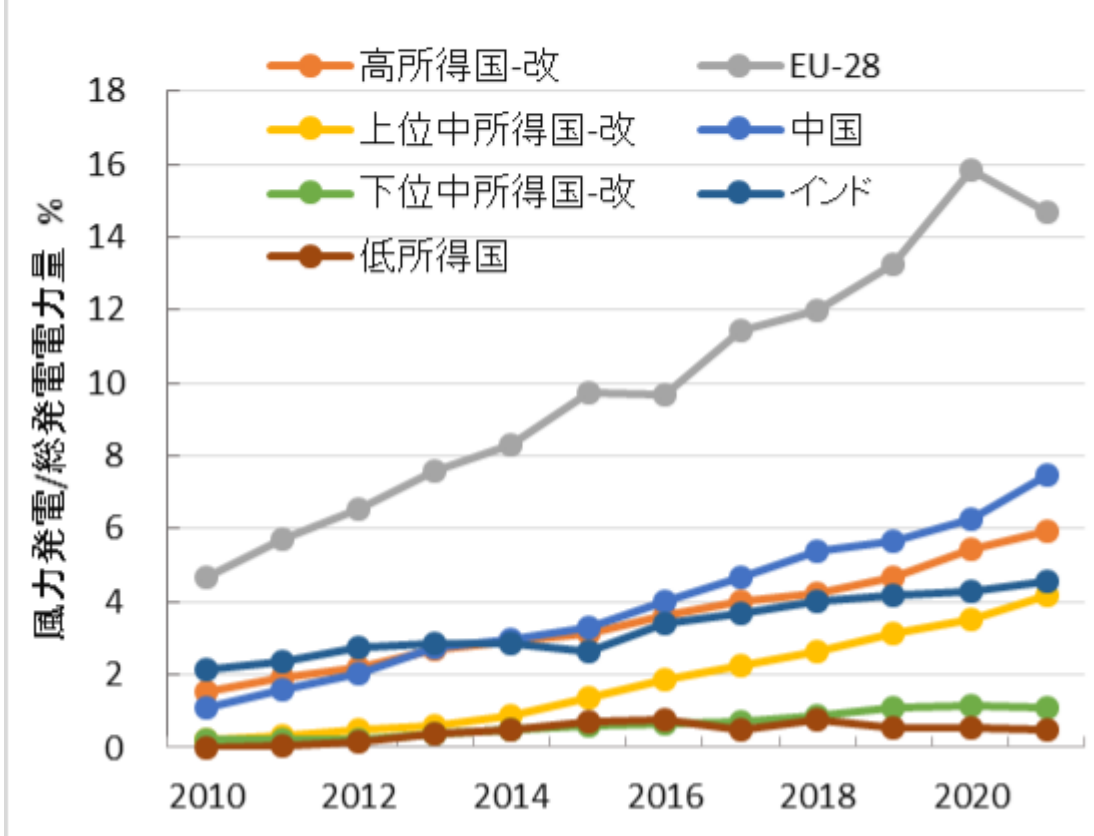
図-14 総発電量に対する風力発電比率の推移 出所: eiaデータで作成
