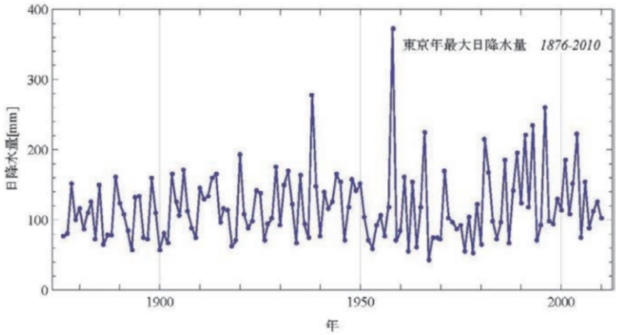
図3-1-4 東京の 1876-2010 の年最大日降水量
