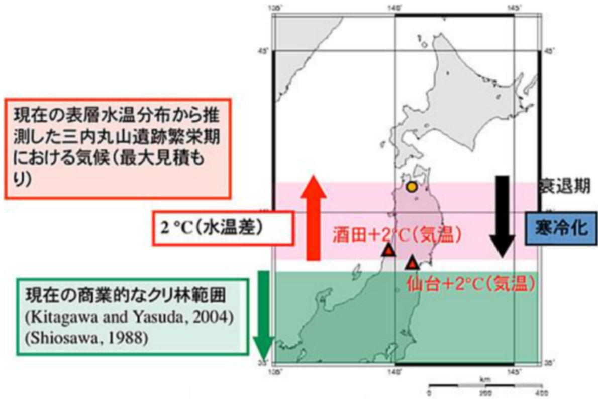
第2図. 2℃という水温、気温差は緯度方向で230kmに相当する。 縄文中期には青森県でも立派な実のなるクリ林があったと考えられる。
