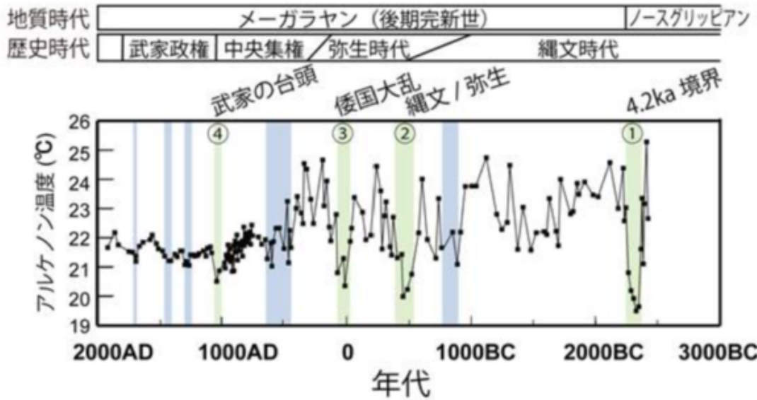
図6：海洋堆積物コアのアルケノン分析から明らかになった、過去4400年間の東京湾の表層水温変動。緑のハッチは特に大きな寒冷化があった時期を示す。
