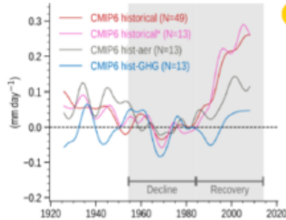
(d) Sahel precipitation anomalies (CMIP6) Baseline period is 1955-1984
