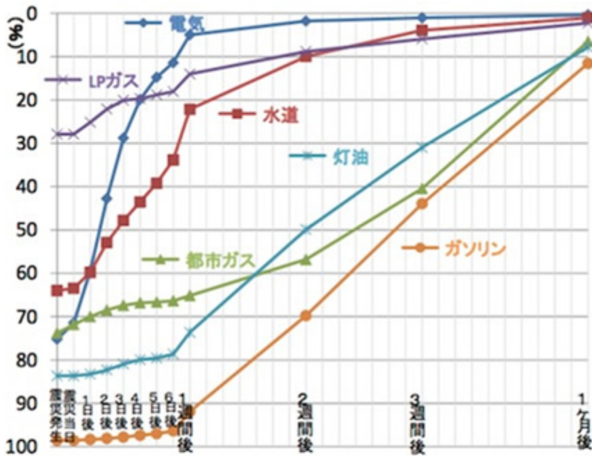
図2 被災三県におけるライフライン途絶率**の推移
