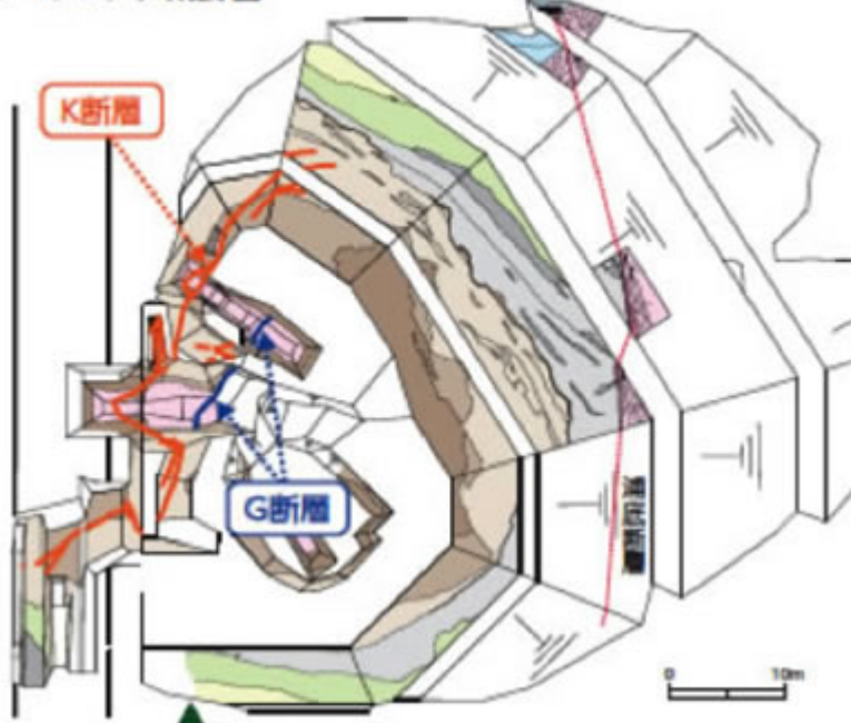
D-1トレンチ概要図
