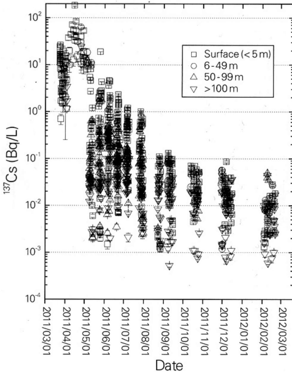
宮城県、福島県および茨城県沖合の海水に含まれる ^{137}\text{Cs} の経時変化 24) 2011年3月～2012年3月。
